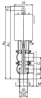
Válvula de conmutación
